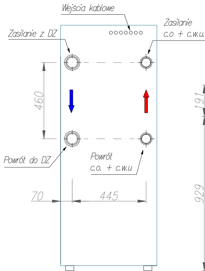
Widok z tyłu PCSY jednomodułowa
