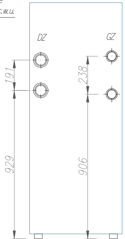
Widok z tyłu PCSY z 3 modułami
