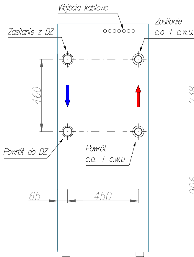
Widok z tyłu PCST jednomodułowa
