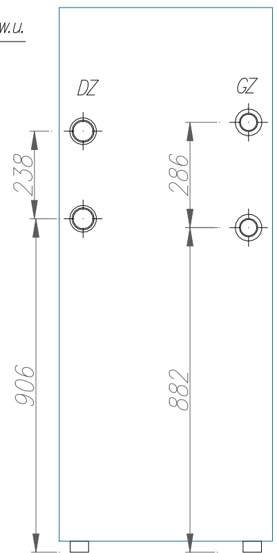
Widok z tyłu PCST z 2 modułami
