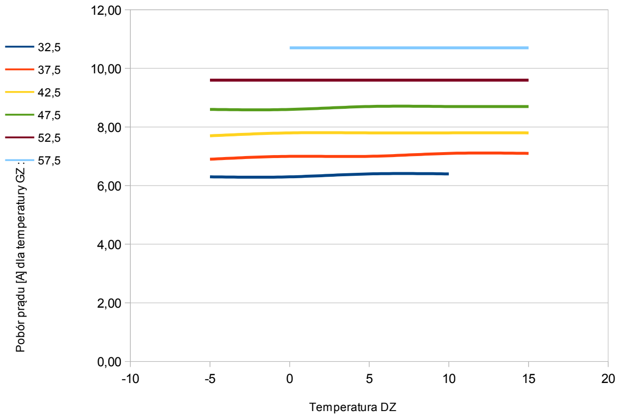
Rys. 4. Pobór prądu przez pompę ciepła PCSK14G
