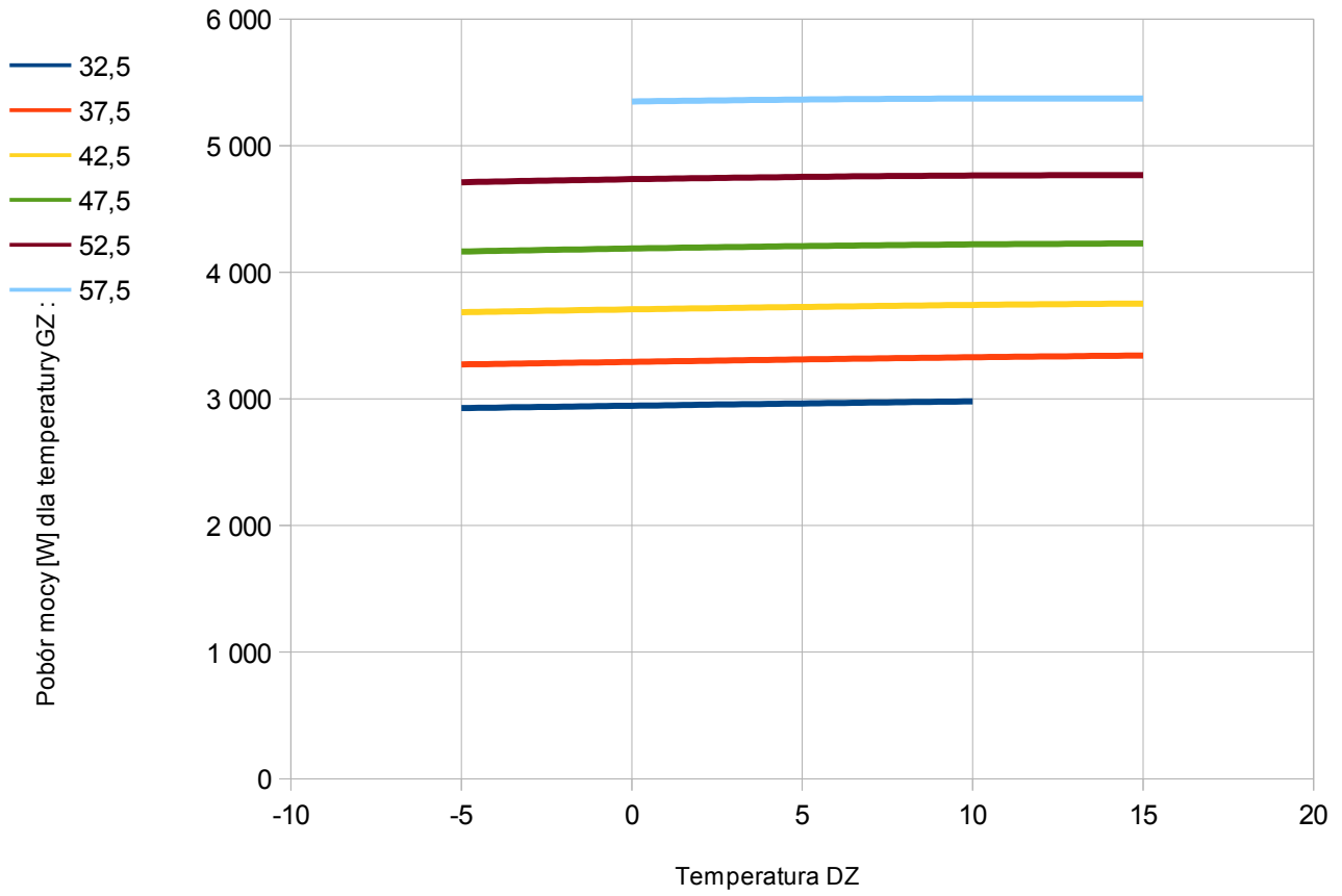
Rys. 3. Pobór mocy elektrycznej przez pompę ciepła PCSK14G
