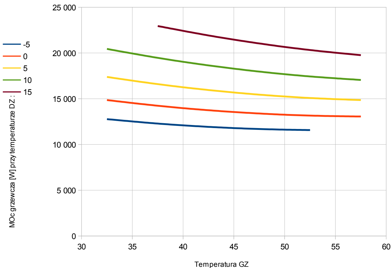
Rys. 1. Moc grzewcza pompy ciepła PCSK14G
