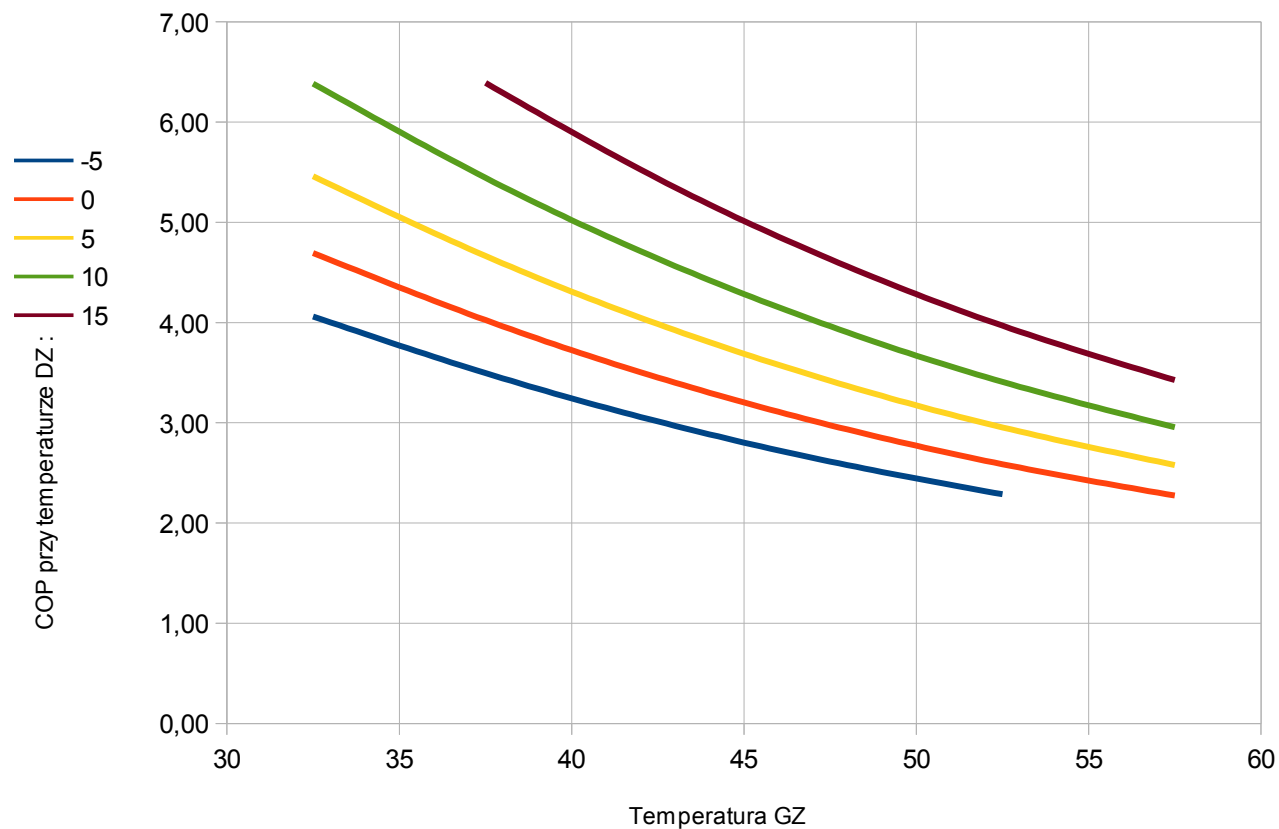
Rys. 2. COP pompy ciepła PCSK14G
