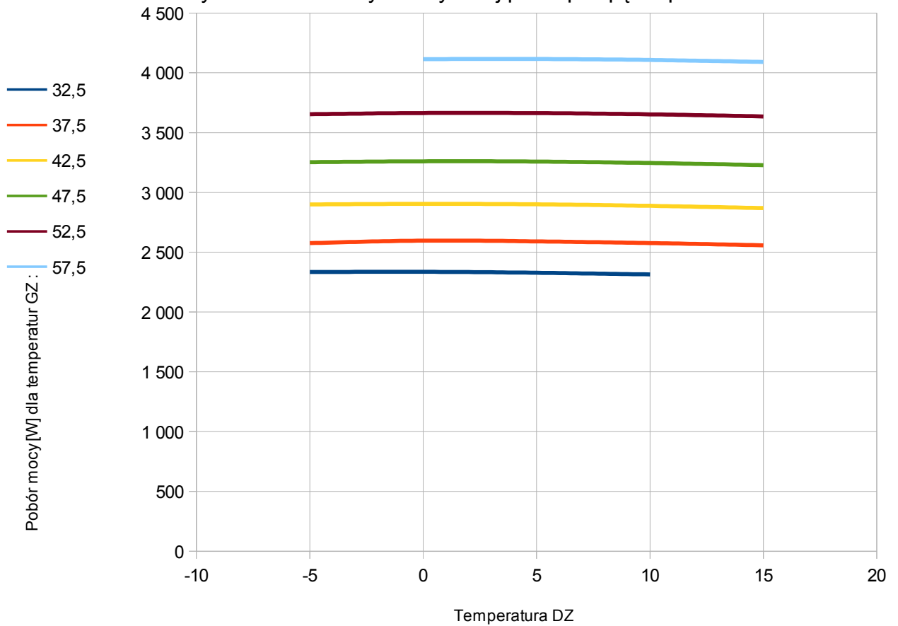
Rys. 3. Pobór mocy elektrycznej przez pompę ciepła PCSK10G
