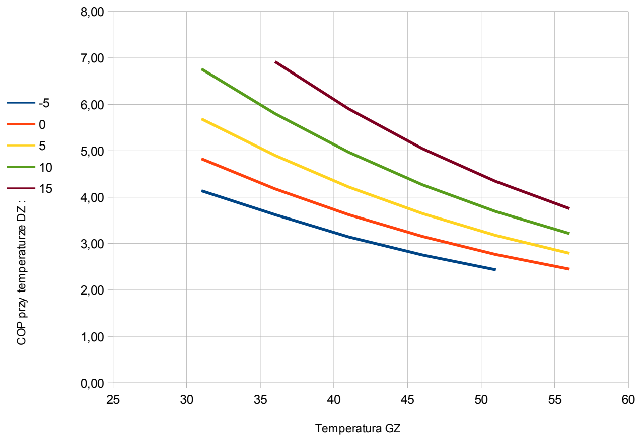
Rys. 2. COP pompy ciepła PCSK10G
