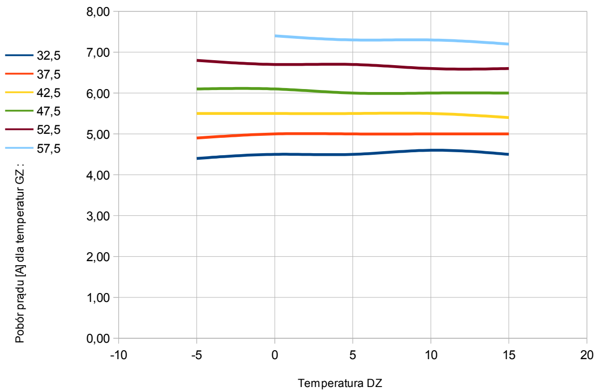
Rys.4. Pobór prądu przez pompę ciepła PCSK10G
