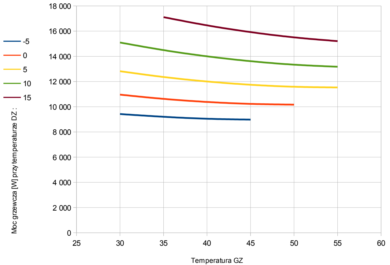
Rys. 1. Moc grzewcza pompy ciepła PCSK10G
