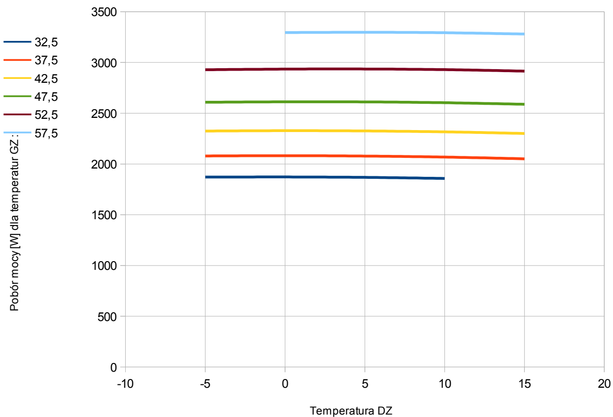
Rys. 3. Pobór mocy elektrycznej przez pompę ciepłą PCSK08G
