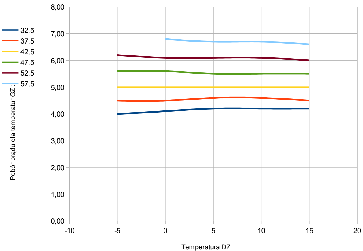
Rys. 4. Pobór prądu przez pompę ciepłą PCSK08G
