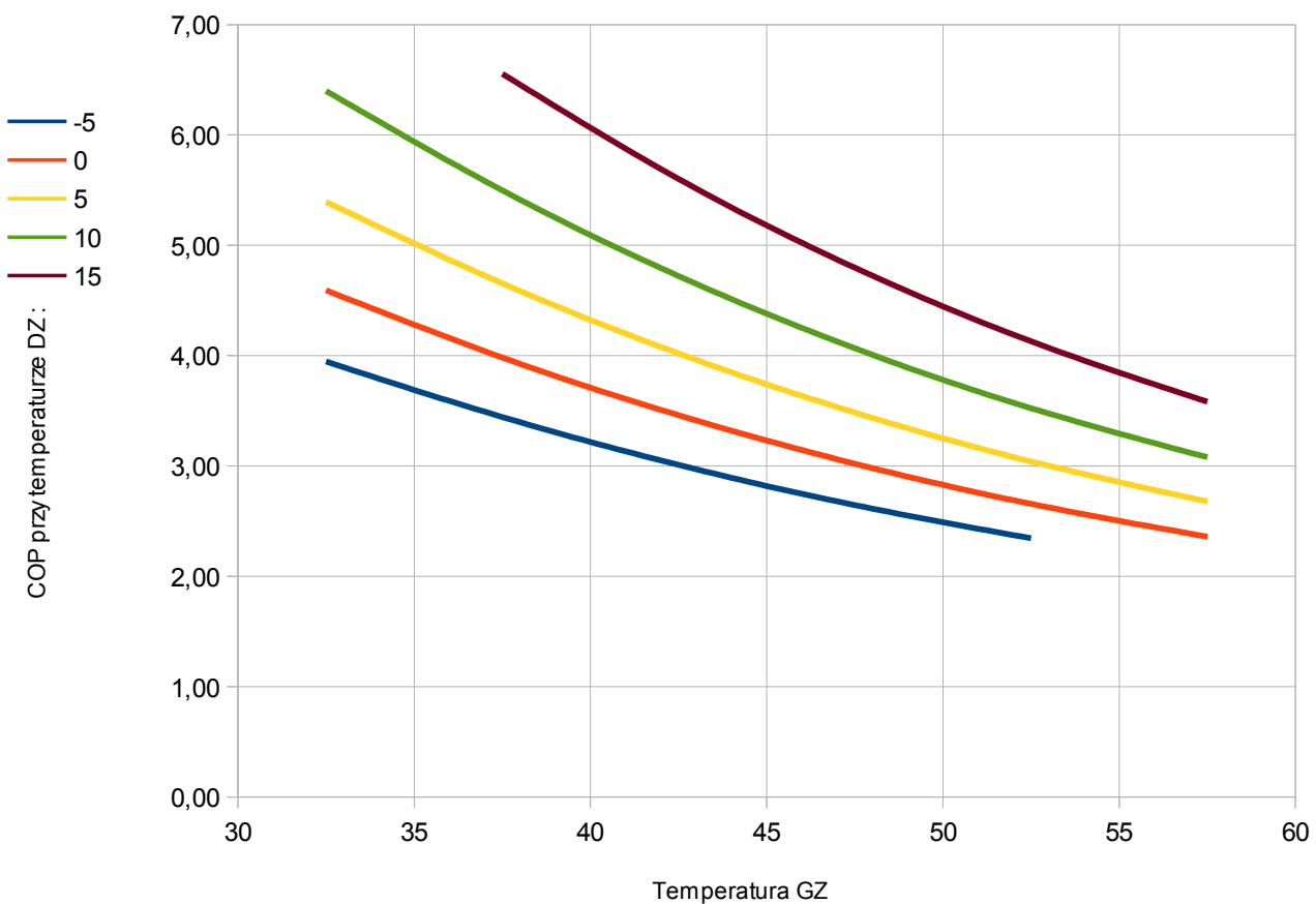
Rys. 2. COP pompy ciepła PCSK08G
