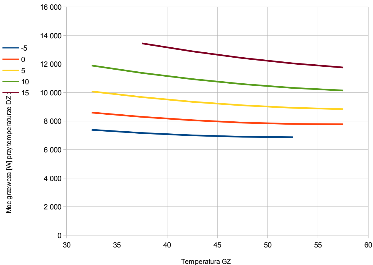
Rys. 1. Moc grzewcza pompy ciepła PCSK08G
