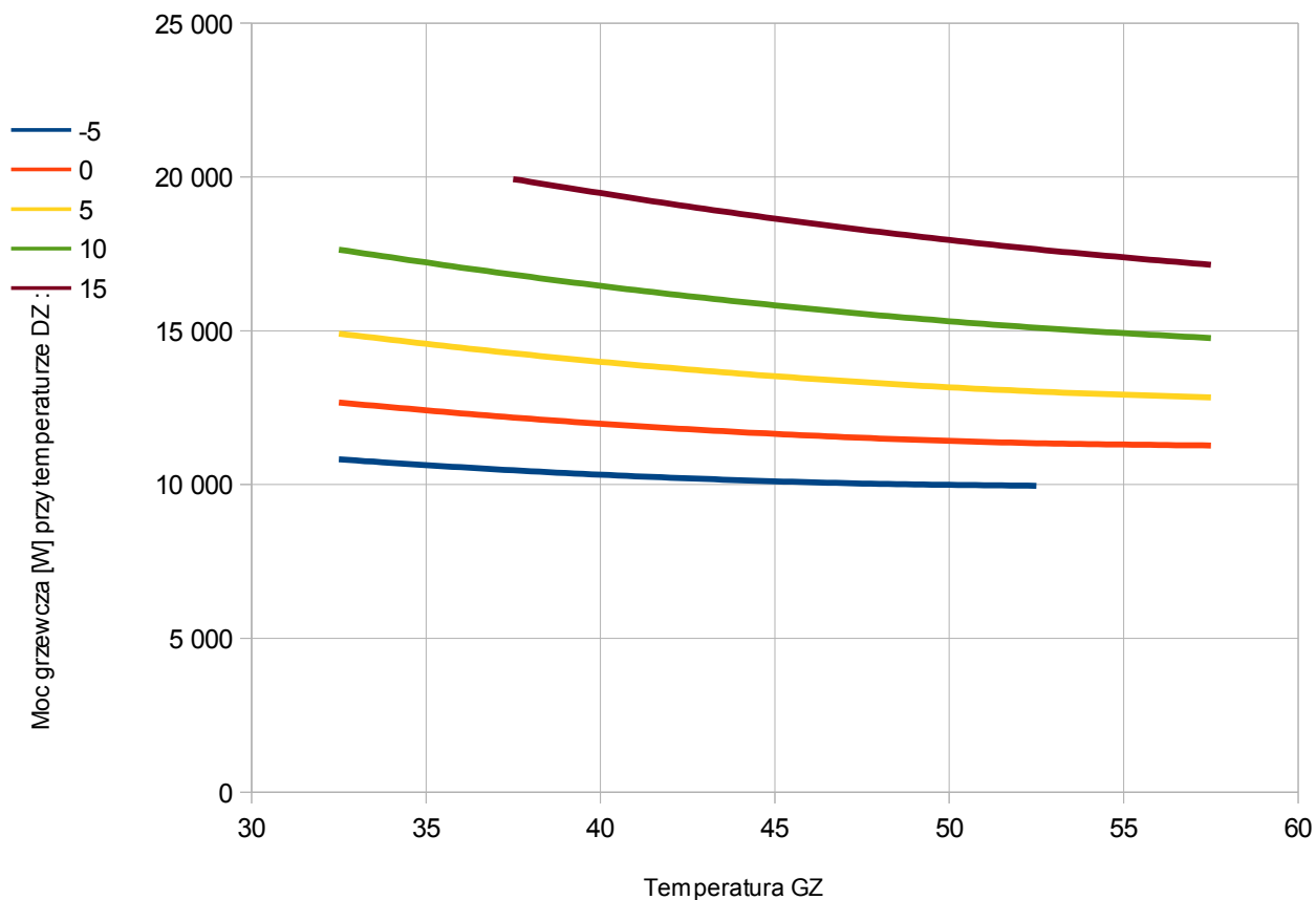
Rys. 1. Moc grzewcza pompy ciepła PCS12G
