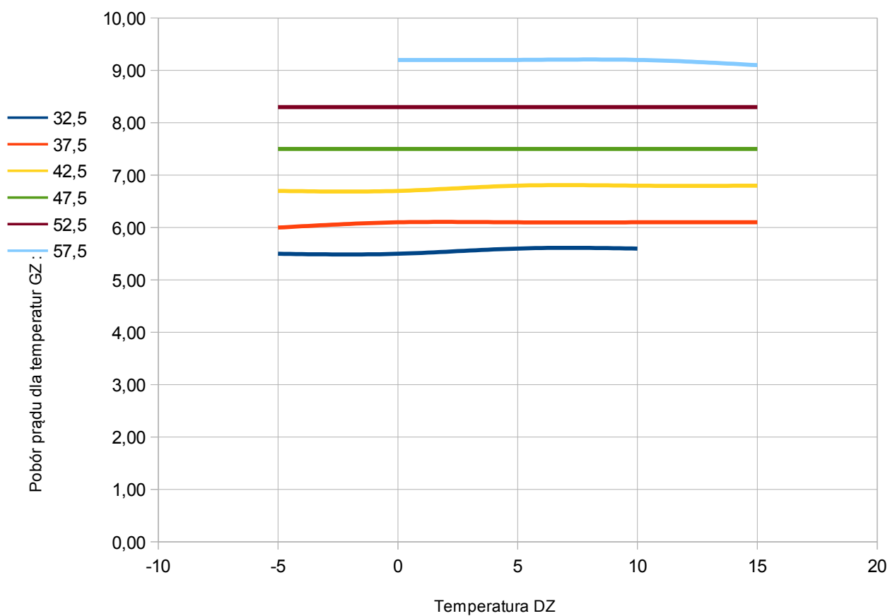
Rys. 4. Pobór prądu przez pompę ciepła PCS12G
