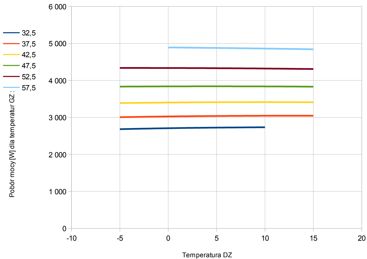
Rys. 3. Pobór mocy elektrycznej przez pompę ciepła PCS12G
