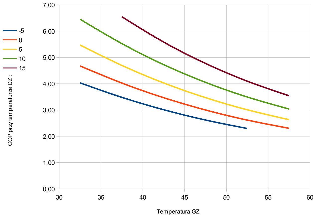
Rys. 2. COP pompy ciepła PCS12G
