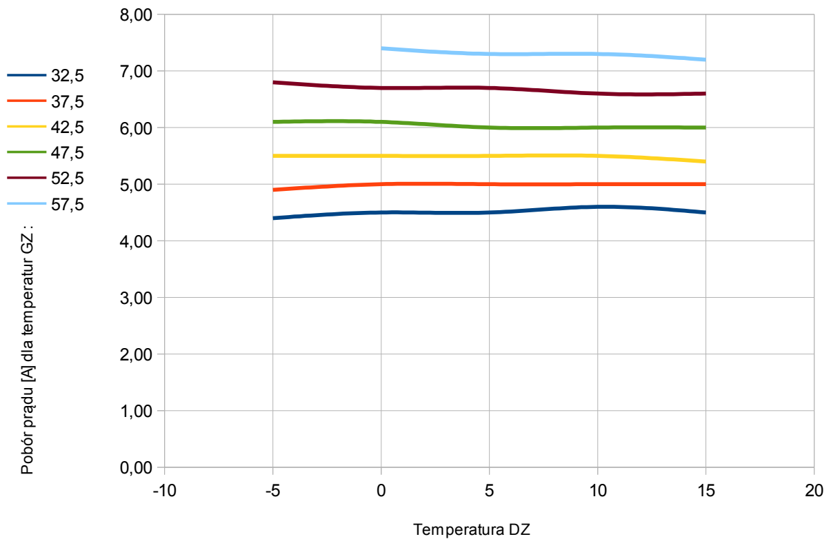
Rys.4. Pobór prądu przez pompę ciepła PCS10G
