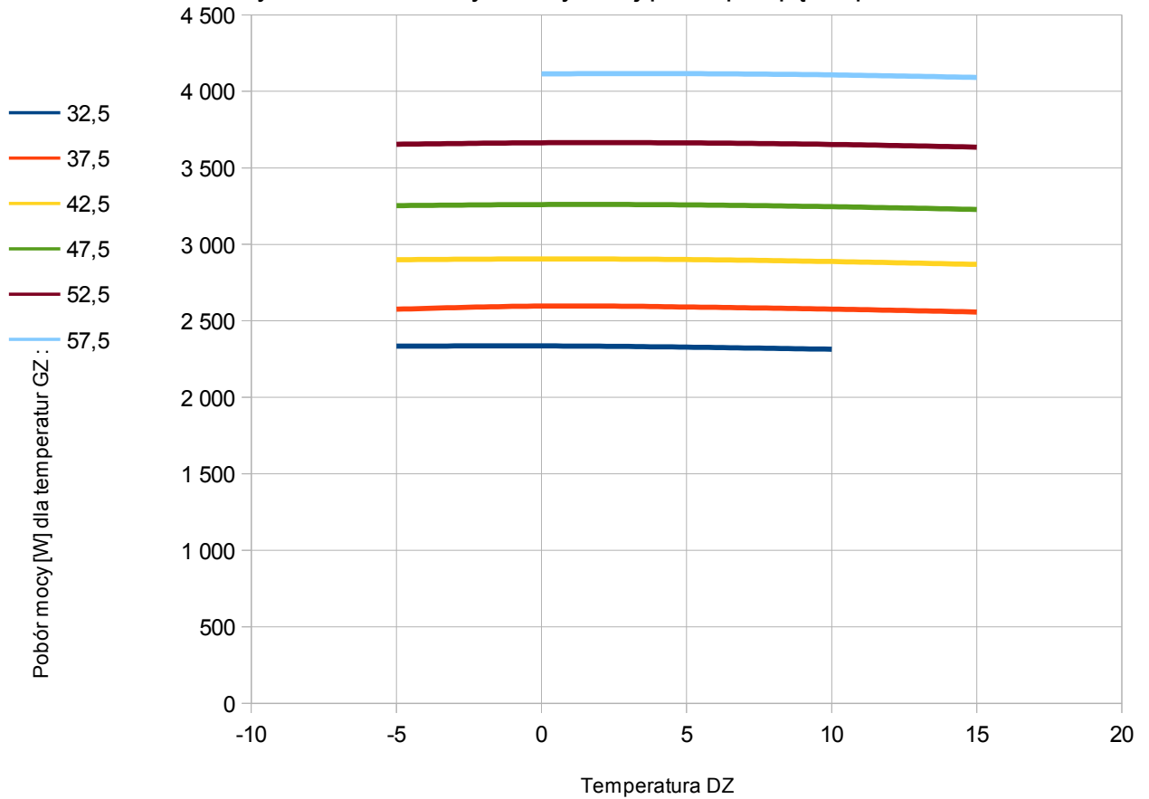
Rys. 3. Pobór mocy elektrycznej przez pompę ciepła PCS10G
