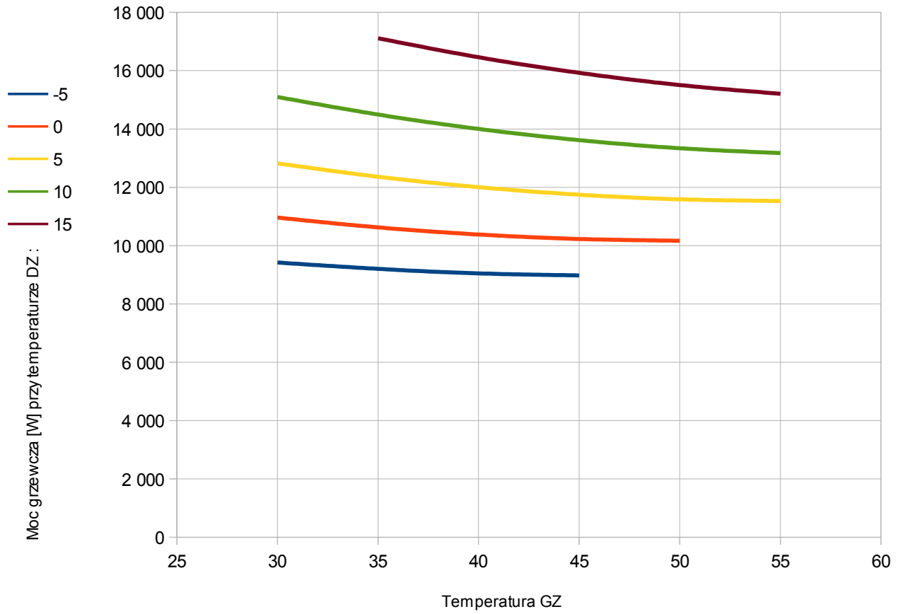
Rys. 1. Moc grzewcza pompy ciepła PCS10G
