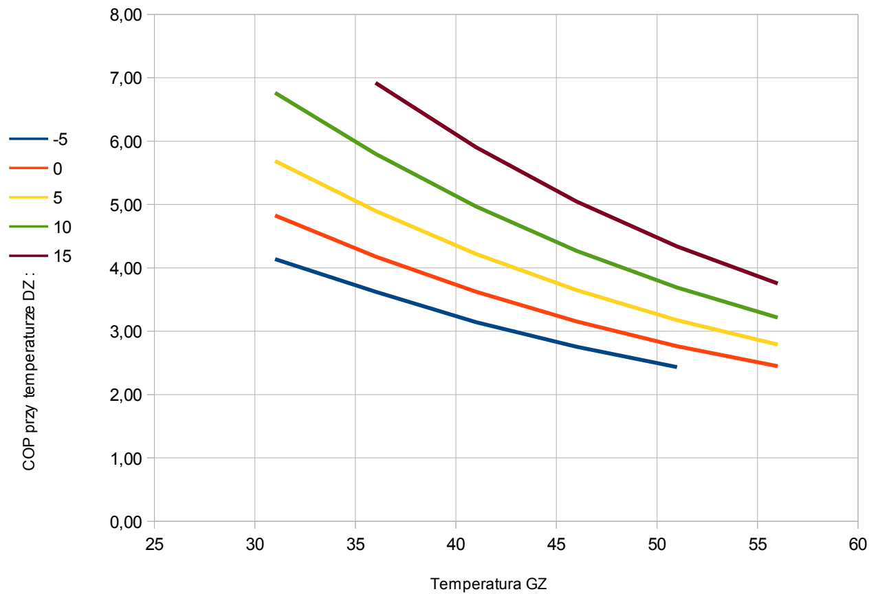
Rys. 2. COP pompy ciepła PCS10G
