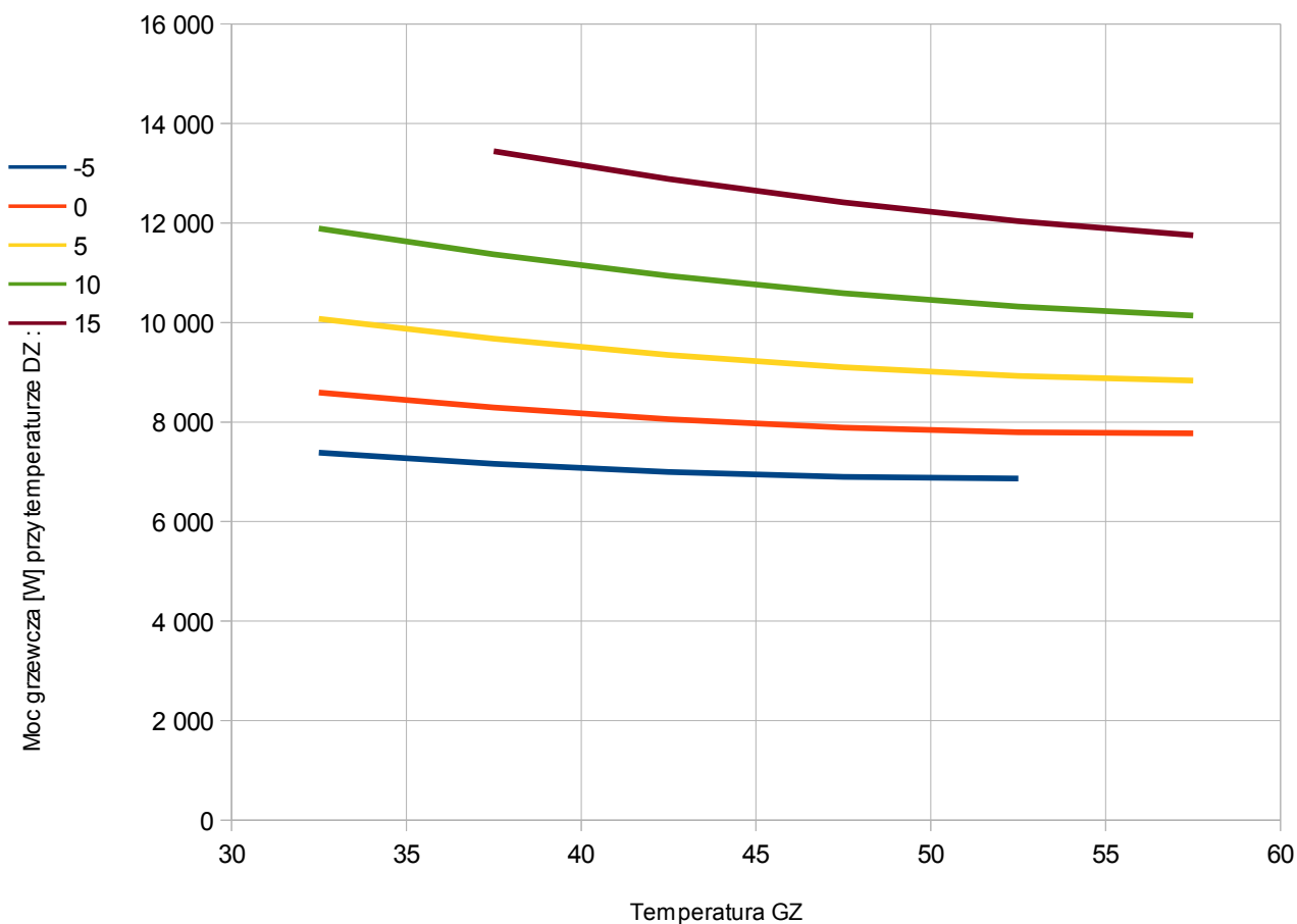
Rys. 1. Moc grzewcza pompy ciepła PCS08G
