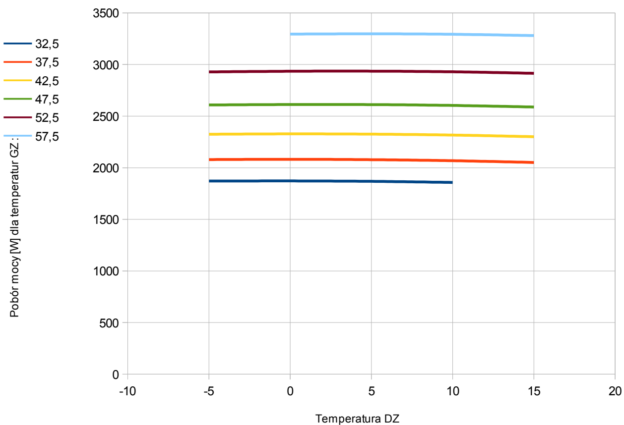
Rys. 3. Pobór mocy elektrycznej przez pompę ciepłą PCS08G
