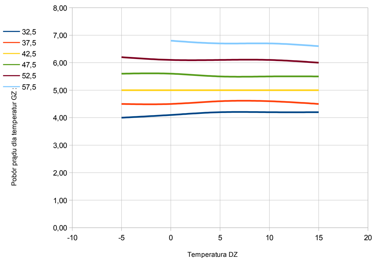
Rys. 4. Pobór prądu przez pompę ciepłą PCS08G
