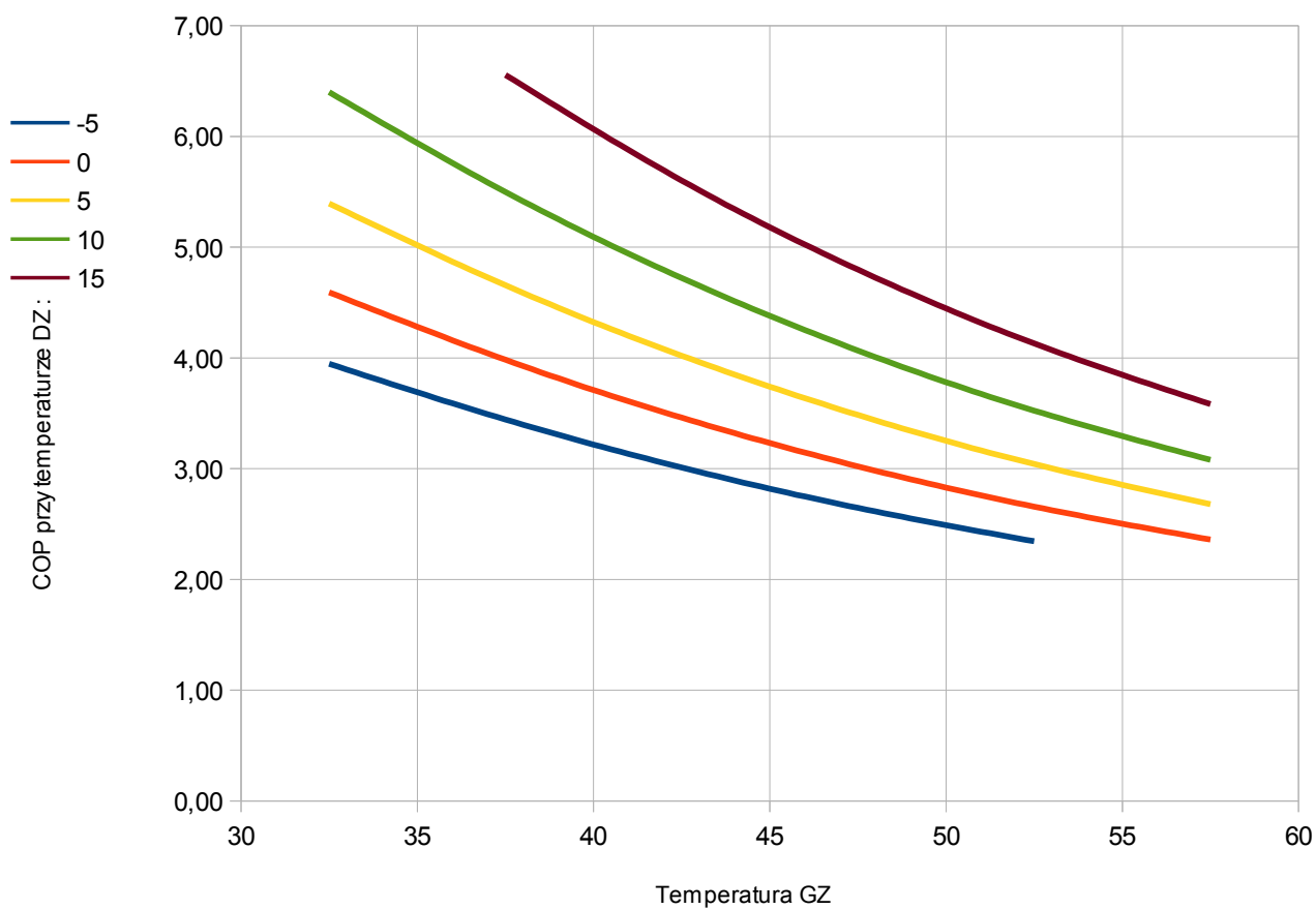
Rys. 2. COP pompy ciepła PCS08G
